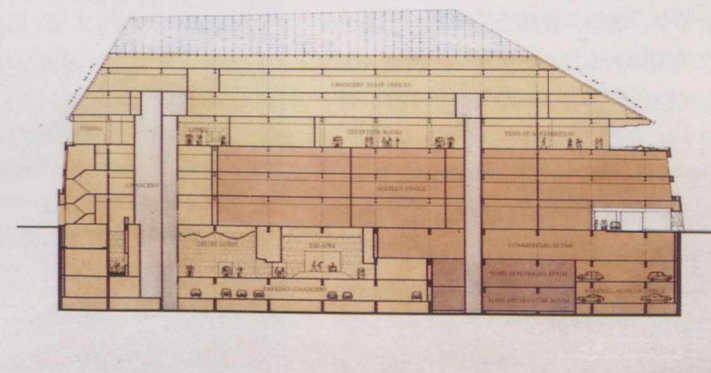
新庁舎の断面図。4階から8階までと地下2階が大使館。1~3階は賃貸部分。駐車場は地下3階にある。
