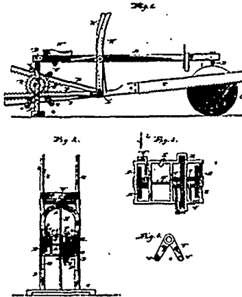
28360 Reichert's Drag Saw.
