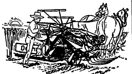
LIEUSE IDEAL DEERING
