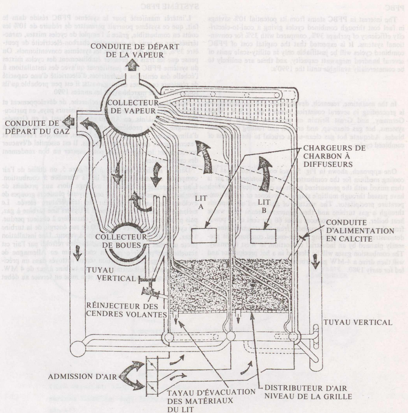
Fig. 4—Coupe de la chaudière à vapeur à lit fluidisé, d'une capacité de 45 tonnes par heure, et installée à l'université de Georgetown (document aimablement transmis par la Foster Wheeler Ltd.)
