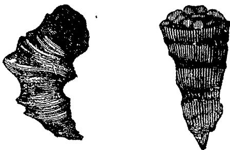
Fig. 16. Cyathophyllum distortum (Hall)
