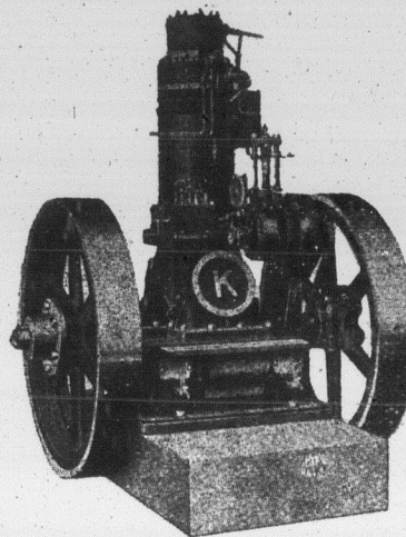
Engin à l'huile brute,
