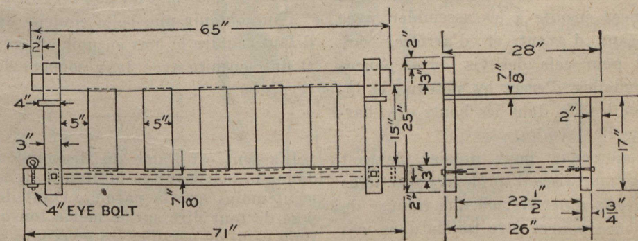
Détails des mesures à prendre pour fabriquer cette balançoire.
