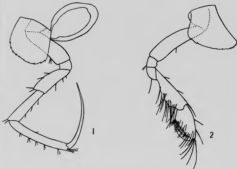
Figure 3. Rozinante fragilis (Goës).
