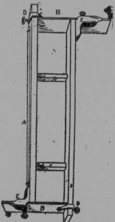
Verstellbare Form für Zaunriegel und Pfosten.
