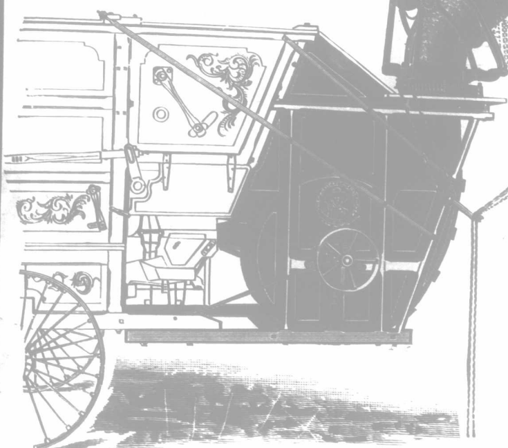
S. &amp; M. Wind Stacker.
