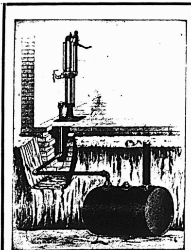
GRAVURE No. 42. POUR GAZOLINE— RÉSERVOIR SOUTERRAIN. POMPE DANS LE BATIMENT.
