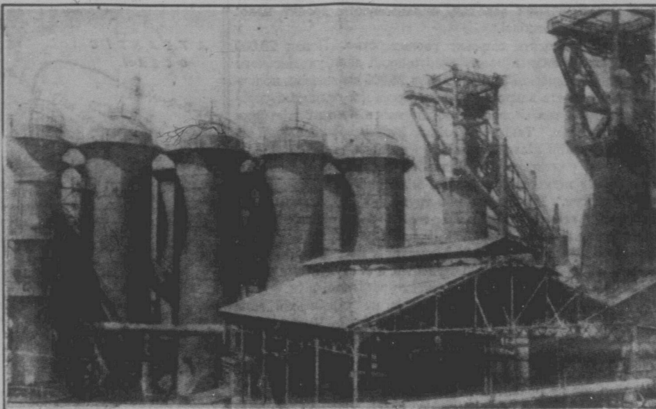
ОДНА З ДОМЕННИХ ПЕЧІВ НОВОЗБУДОВАНОГО МЕТАЛУРГІЙНОГО ЗАВОДУ В КЕРЧІ. ЦЯ ДОМНА ВИТОПЛЮЄ 500 ТОН ЧАВУНУ НА ДОБУ.
