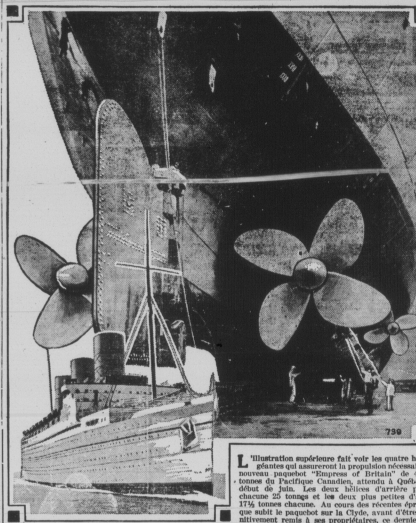
L'illustration supérieure fait voir les quatre hélices géantes qui assureront la propulsion nécessaire au nouveau paquebot "Empress of Britain" de 42,500 tonnes du Pacifique Canadien, attendu à Québec au début de juin. Les deux hélices d'arrière pesent chacune 25 tonnes et les deux plus petites d'avant 17½ tonnes chacune. Au cours des récentes épreuves que subit le paquebot sur la Clyde, avant d'être définitivement remis à ses propriétaires, ce dernier put atteindre une vitesse maximum de 25½ nœuds sur le mille mesuré. — On peut aussi voir sur la gravure le puissant gouvernail du super-paquebot, qui pèse 67 tonnes. Pour transporter ce gouvernail sur les chantiers maritimes, il fallut se servir d'un camion spécialement construit à cet effet et quelques jours auparavant, une équipe d'hommes avait libéré la route des poteaux de téléphone et autres obstacles qui auraient pu entraver son passage.
