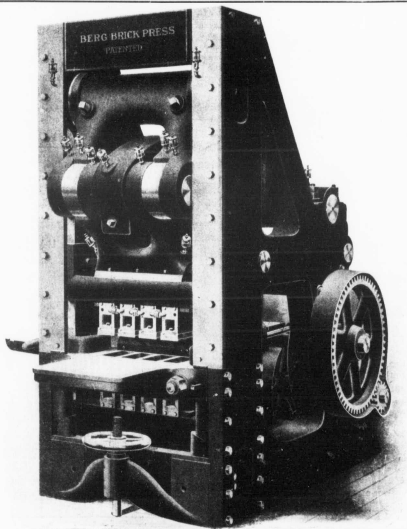
IMPROVED BERG BRICK PRESS
