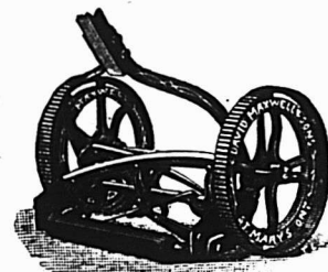
LA TONDEUSE A GAZON "THE MAXWELL" AVEC ROUE DE 10 p.c.
