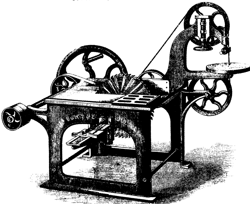
POWIS & CO., PATENT SAWING MACHINE.
