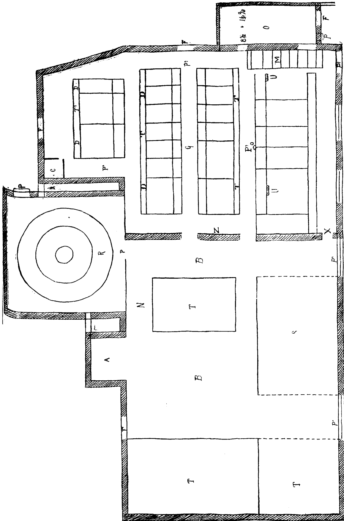
Planche VI.—Bâtiment de Messieurs Ignace et Jules N. Paquet, de St-Nicolas, Q., (suite).—Plan par terre.—Légende.
