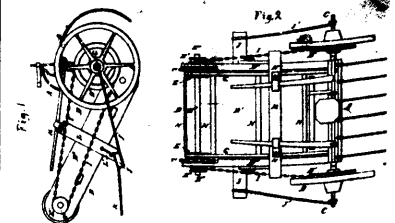
6464 Williams' Hay Loader.
