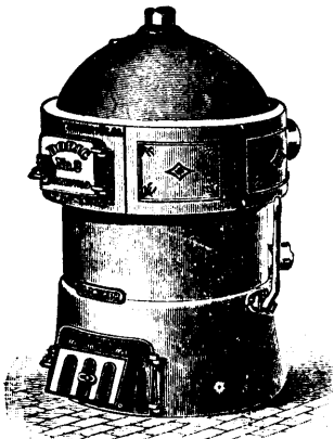
(Complete Boiler.)
