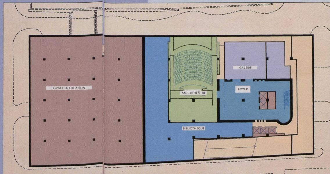
Plan du 2ème sous-sol
