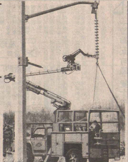
架線機械人
