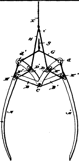
83223 Lucky's Hay Fork.
