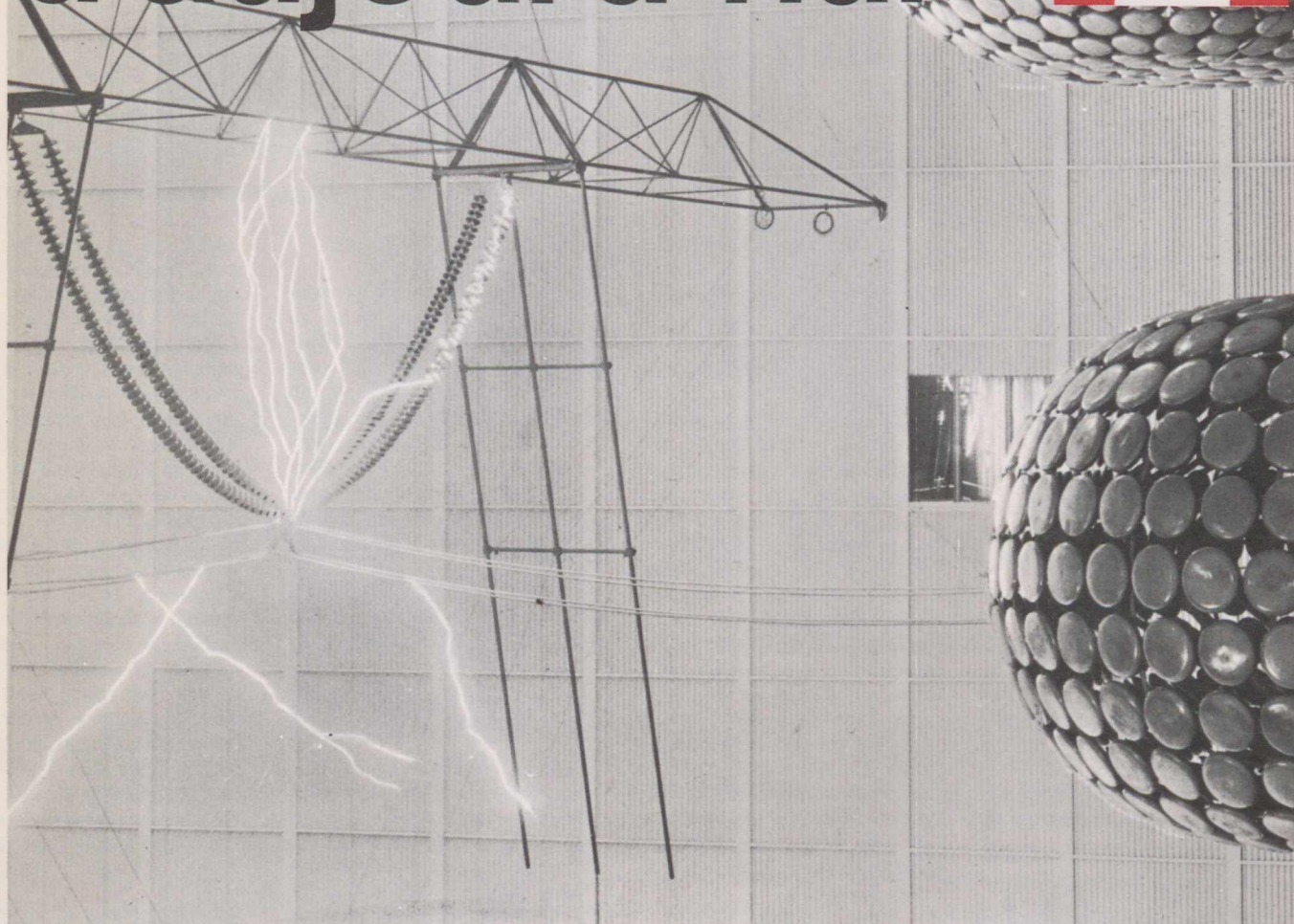
Dans le laboratoire haute tension de l'Institut de recherche de l'Hydro-Québec.
