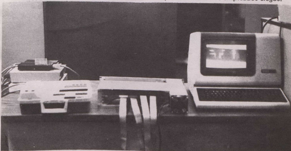
Material utilizado para el experimento: la máquina VersaBraille (a la derecha), la caja negra o vinculadora (en el centro) y la terminal RAPID (a la izquierda).
