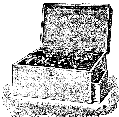
Type d'appareil à l'aradisation à 4 éléments avec rhéostat.
