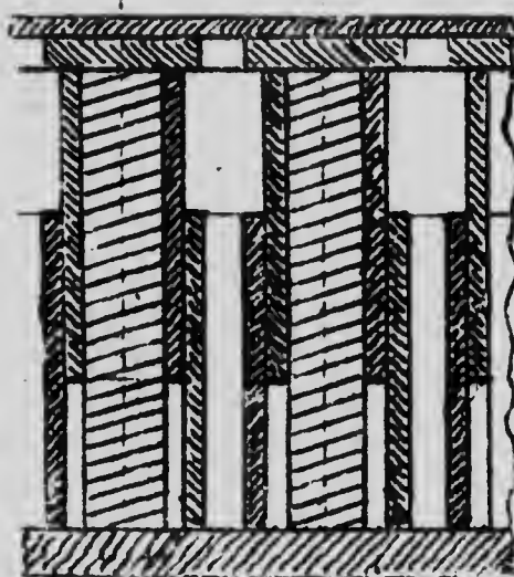
COUTE VERTICALE LONGITUDINALE D'UNE PARTIE DE L'ETRAVE DE VAISSEAU, MONTRANT DEUX DES COUSSINETS A RESSORT.
