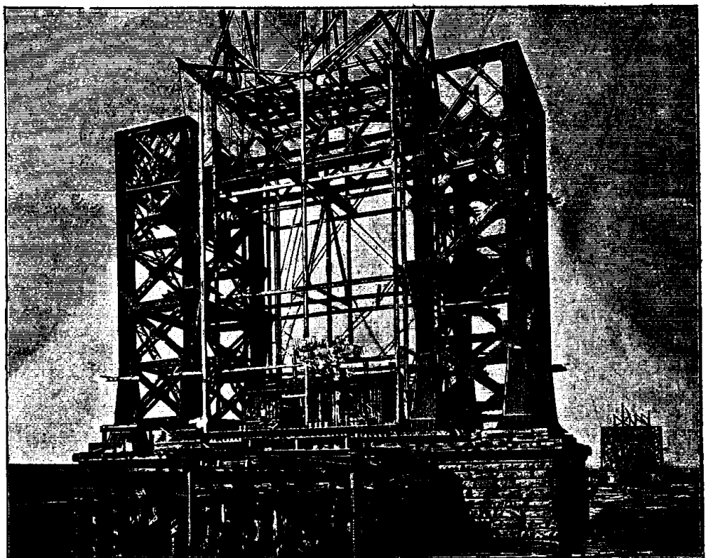
LE NOUVEAU PONT SUSPENDU DE NEW-YORK. — ÉTAT ACTUEL DU MONTAGE DES PIÈCES
