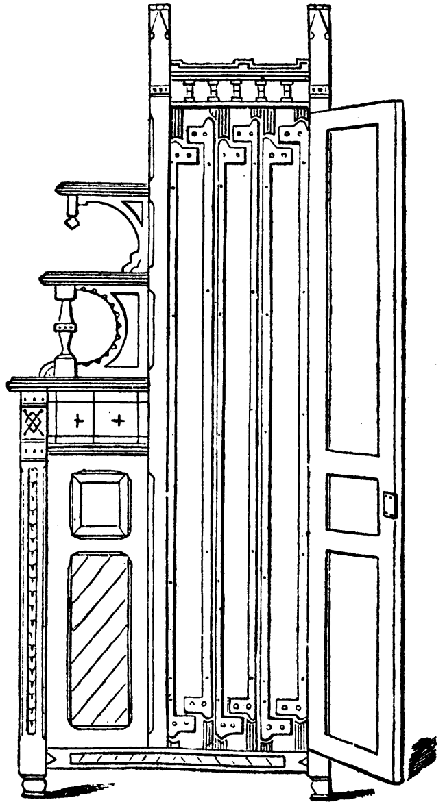
END ELEVATION
