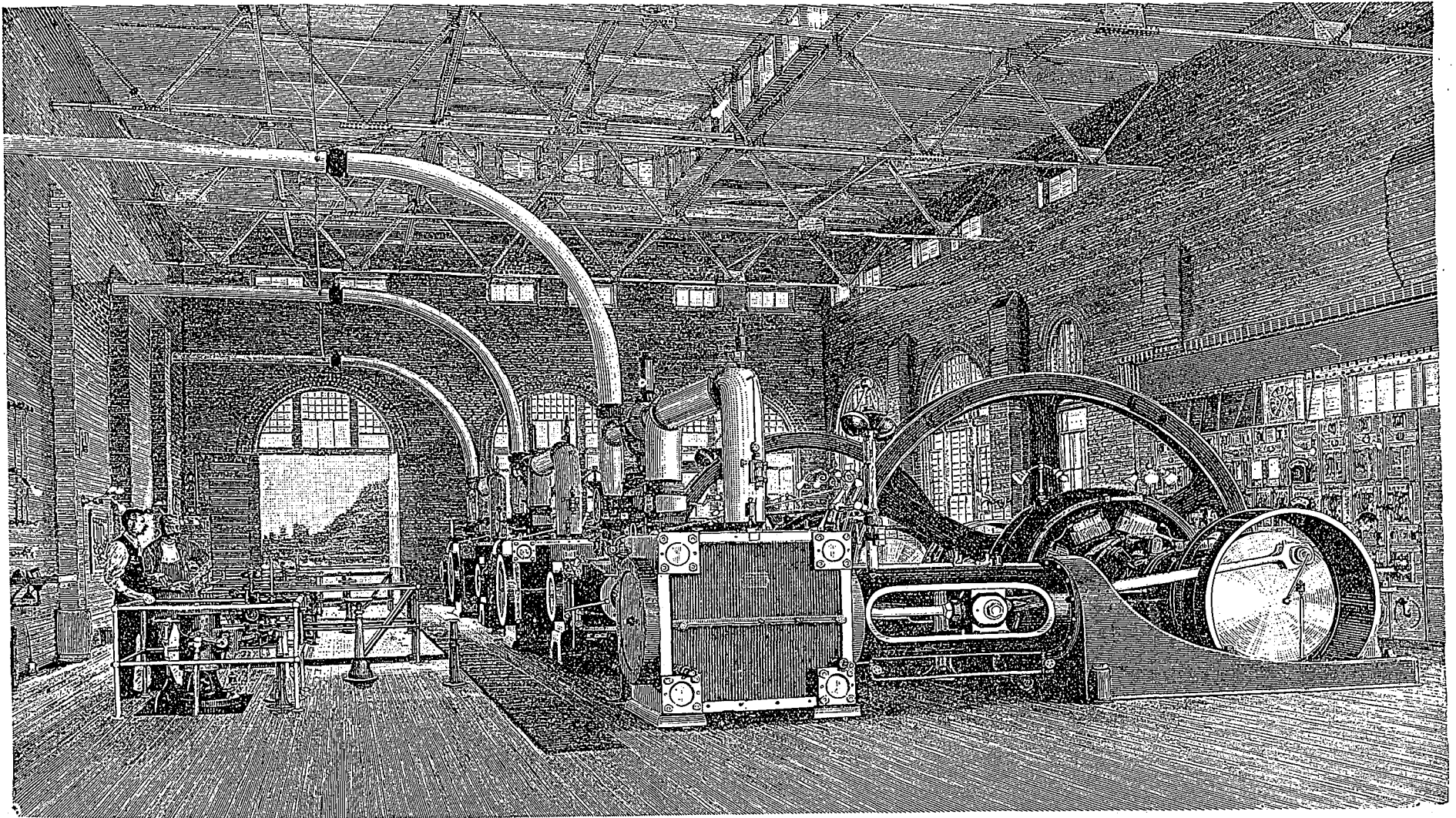
Intérieur d'une Usine fournissant l'électricité aux Chars Urbains.
