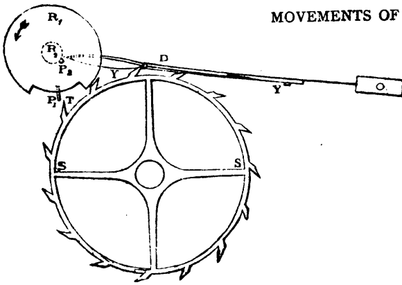
FIG. 21.—Chronometer Escapement.
