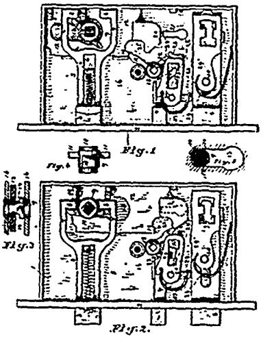
24389 Perkins' Door Lock.
