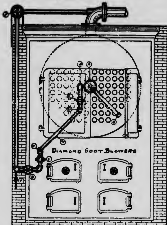
Souffleur à Suie "Diamond", modèle F. installé sur une chaudière horizontale tubulaire.
