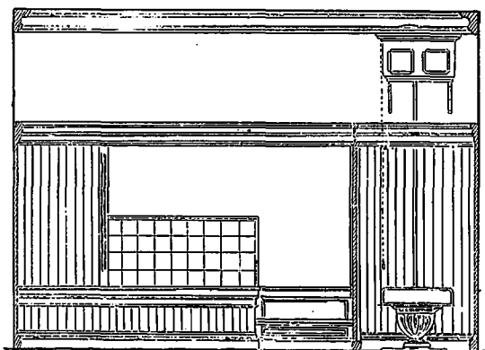
Longitudinal Section
