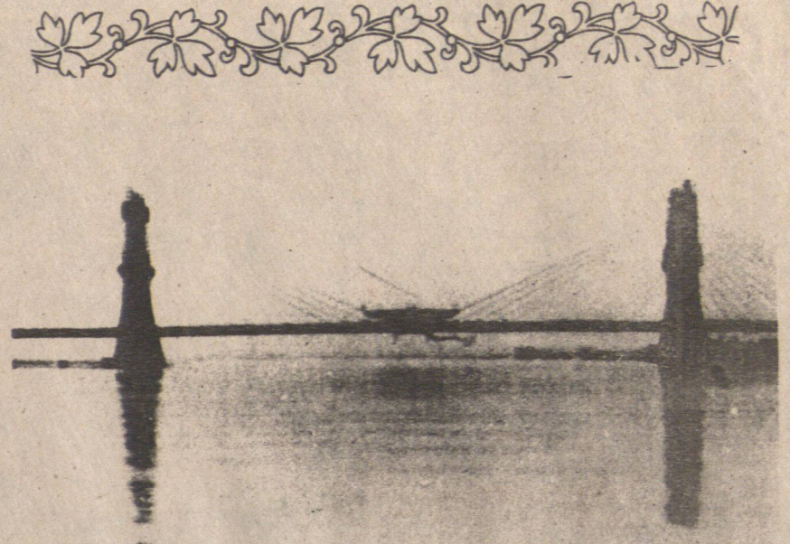
南寧的經路大最洲亞和國中前目 這，龍合日六月二十於橋大路公河黃 四游下口渡口洛郊北南濟在落座它，的工施計設已自國中是，橋大式拉斜力應預座 (片照真傳社華新) •米〇二二速徑跨大最，米八・二二〇二長全，處里公
