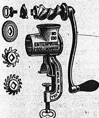
Hache-Viandes "ENTERPRISE," montrant les parties détachées.
