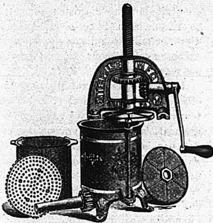
"Stuffer" ou Presse à Saindoux "ENTERPRISE."
