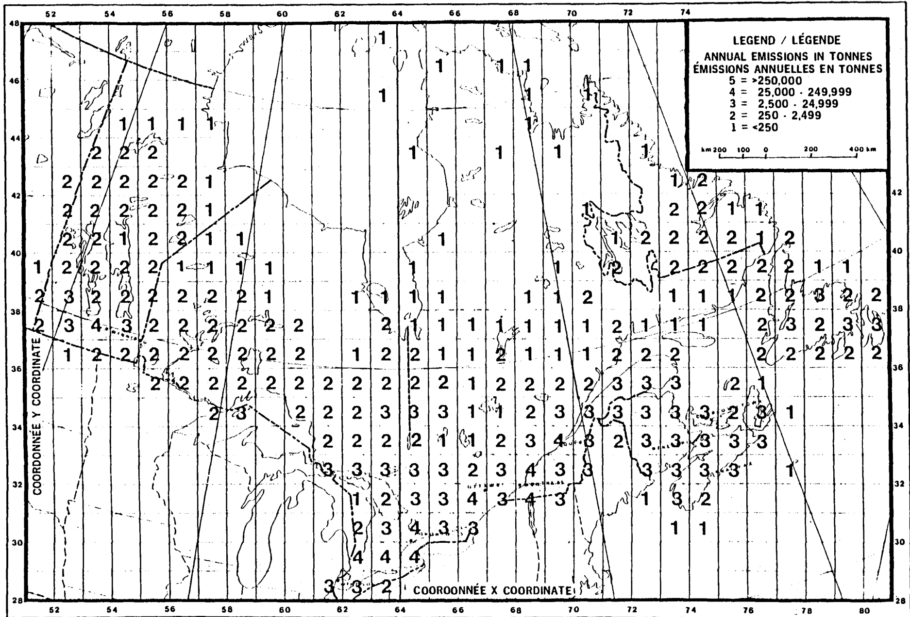
MAGNITUDE AND DISTRIBUTION OF EASTERN CANADA \text{NO}_x (EXPRESSED AS \text{NO}_2 ) EMISSIONS - 1976 DATA BASE ON 127 km x 127 km GRID IMPORTANCE ET RÉPARTITION DES ÉMISSIONS DE \text{NO}_x (EXPRIMÉES EN \text{NO}_2 ) DANS L'EST DU CANADA - DONNÉES DE 1976 SUR GRILLE DE 127 km x 127 km
