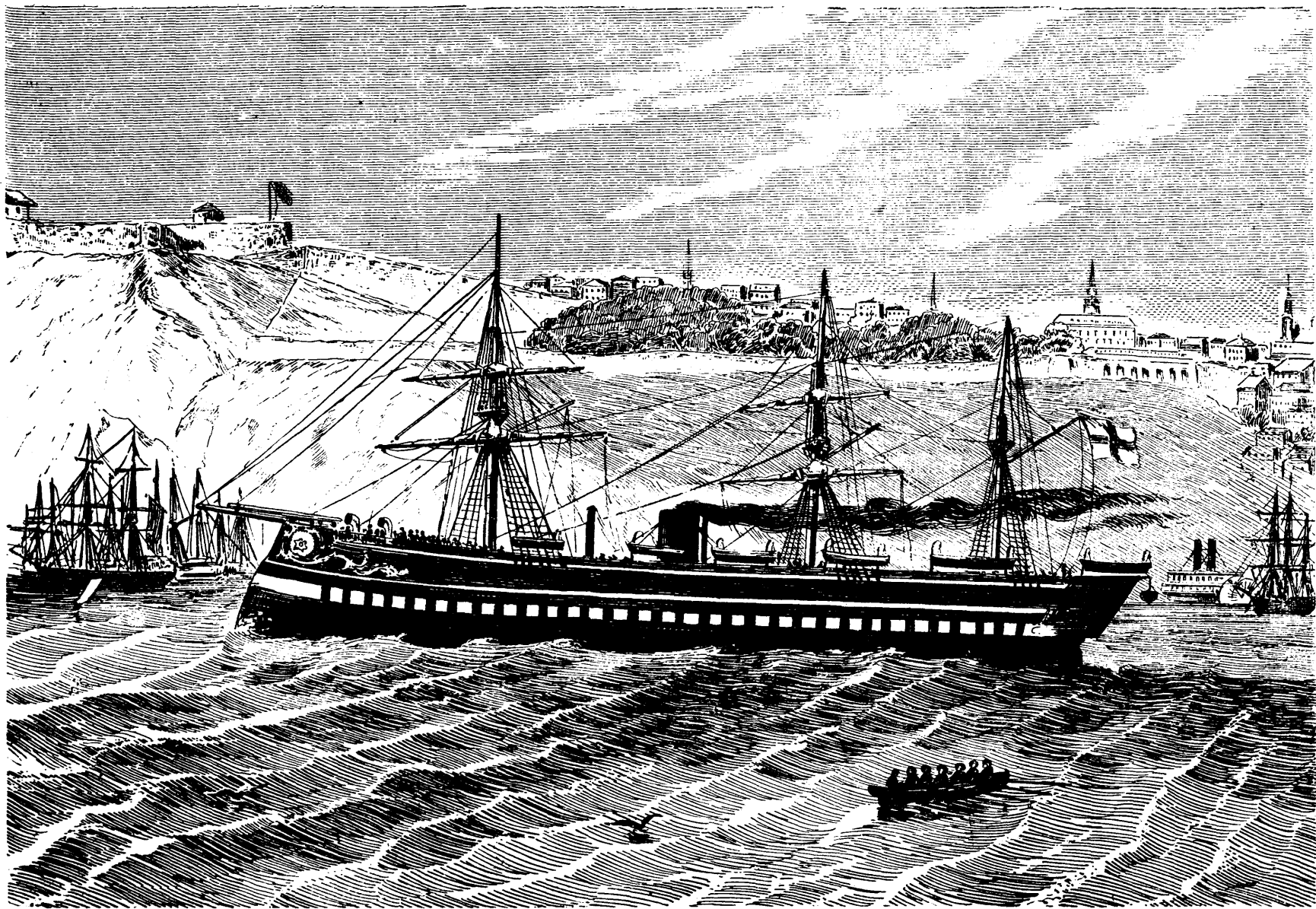
LE NAVIRE A VAPEUR "CROCODILE" DEVANT QUEBEC.—D'après un croquis de W. Carlisle —VOIR PAGE 235.
