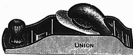
Rabot debout "UNION" No 137. Ce Rabot, tel qu'indiqué dans la gravure ci-dessus, est reversible; il est pourvu de deux lumières et de deux assises par la lame. No 137, longueur 8 pouces, lame 1 1/2 pouces.
