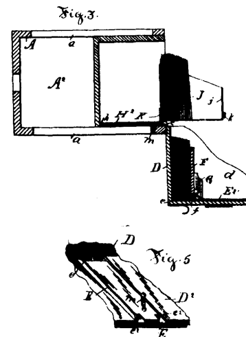
38024 Des Rivieres and Prud'homme's File.
